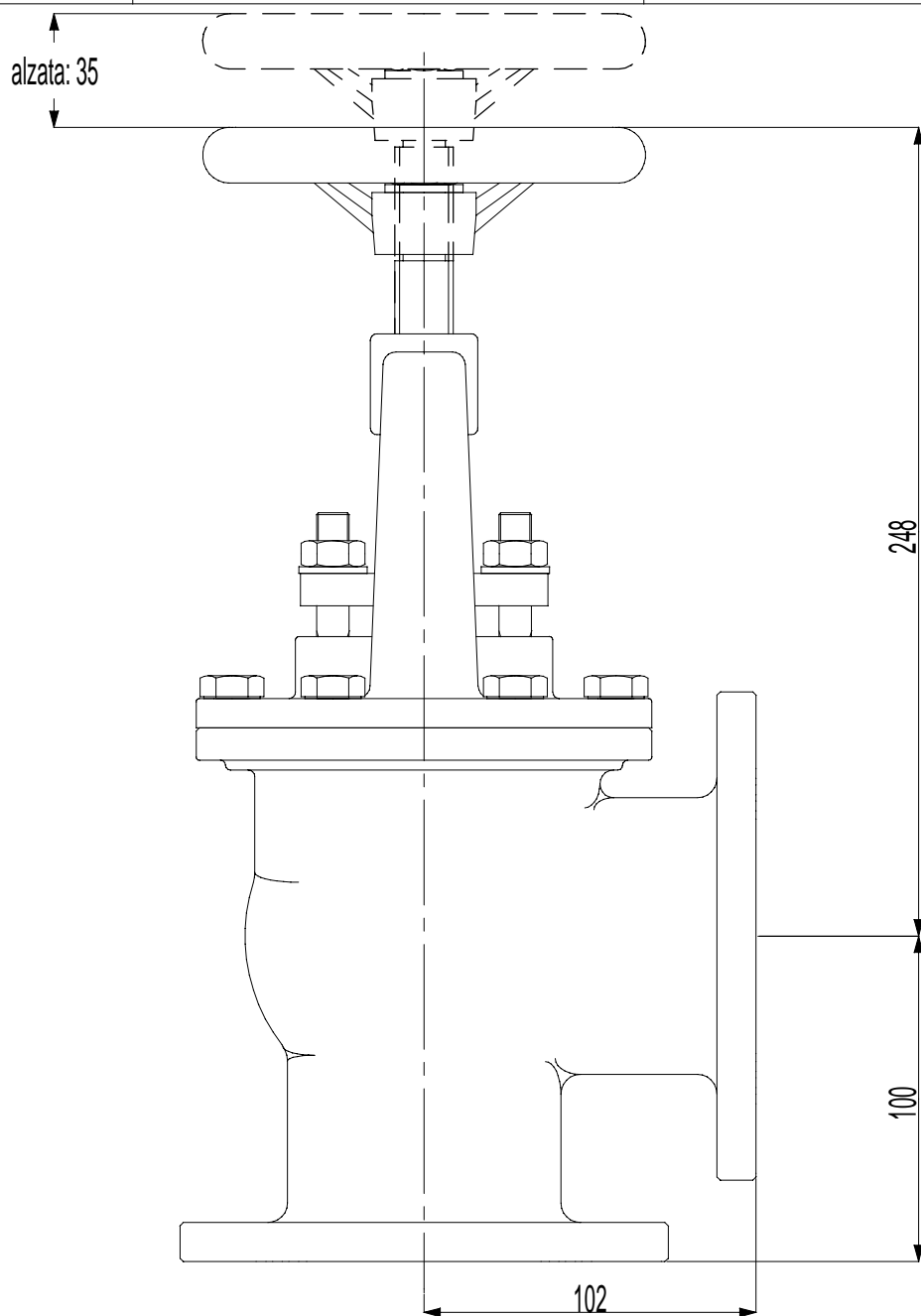
Dimensioni flange
