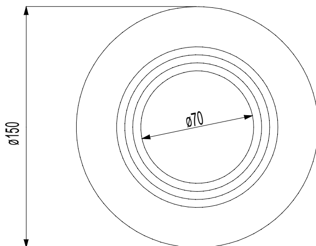
Dimensioni flange
