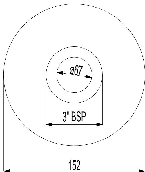
Dimensioni flangia su canotto
