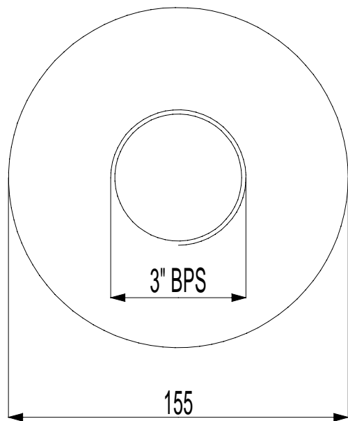
Dimensioni flangia di serraggio
