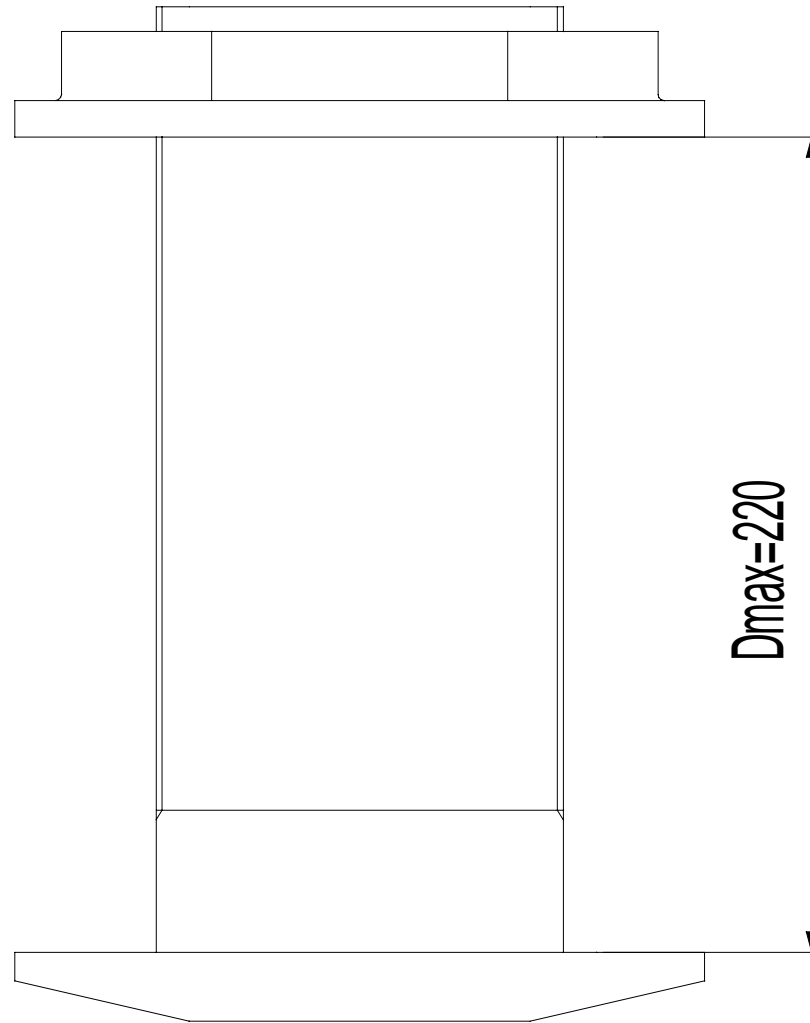
Dimensioni flangia su canotto
