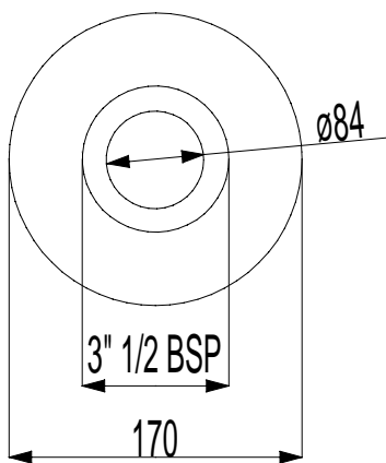
Dimensioni flangia su canotto
