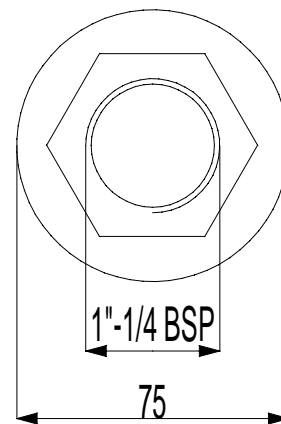
Dimensioni dado di serraggio
