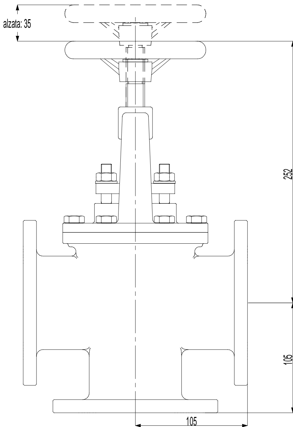
Dimensioni flange
