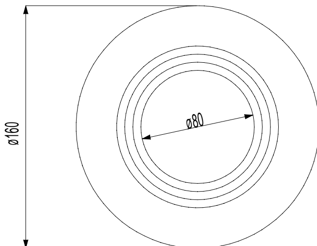
Dimensioni flange
